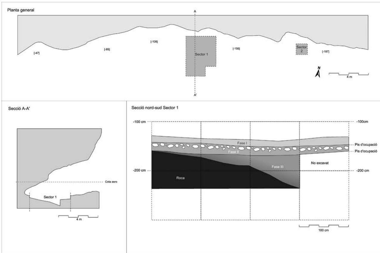
Figura 2. Planta general amb indicació dels sectors d'excavació i seccions.
