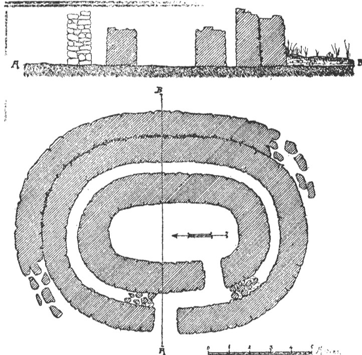
Fig. 12.-Secció i planta de la torre ibèrica de Los Foyos (Lluçena del Cid)
