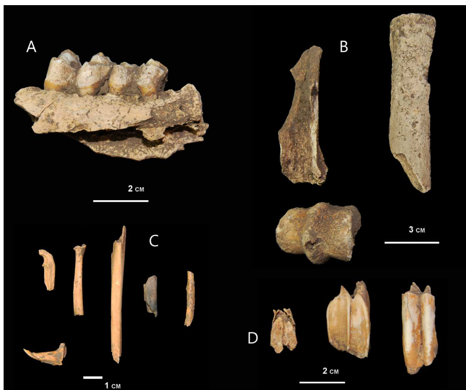
Figura 10. Algunos elementos óseos determinados recuperados. A: mandíbula de Cervus elaphus ; B: fragmentos de un metacarpo de Equus ferus ; C: diversos elementos atribuibles a Oryctolagus cuniculus ; D: piezas dentales aisladas de Capra pyrenaica .
