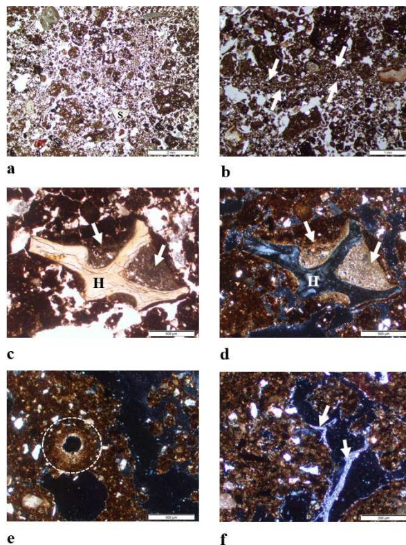
Fig. 3. Micrografías del nivel IIa (Mesolítico reciente). (a) Microestructura migajosa. Se observa un fragmento de sílex (S) en la masa basal en LPP. (b) Costra sedimentaria señalada con flechas en LPP. (c) Fragmento óseo (H) en el cual aparecen residuos cenicientos señalados con flechas en LPP. (d) Igual que la micrografía c pero en LPX. (e) Hipo-revestimiento calcítico en un hueso señalado con un círculo en LPX. (f) Relleno suelto discontinuo de calcita acicular en un hueso señalado con flechas en LPX.
